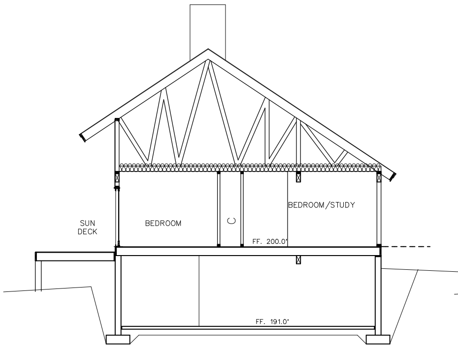
D-D SECTION
